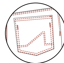
Détail de surpiqûres poche dos
